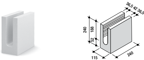
• 4 DF (Breite 115)
