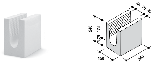
• 5 DF (Breite 150)
